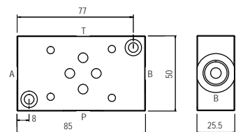
Top & Side Views - G342/01-SE
