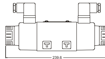
Side View - 110 / 240 Volt AC DFA-03-...-AC...-L-35 Series
