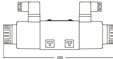
Side View - 110 / 240 Volt AC DFA-03-...-AC...-L-35 Series
