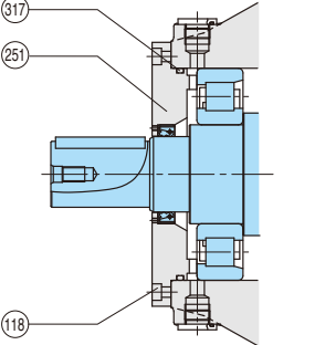
LXV500の場合 in case of LXV500
