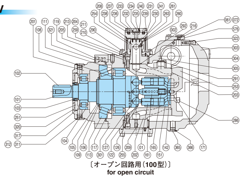
LZV500の場合 in case of LZV500
